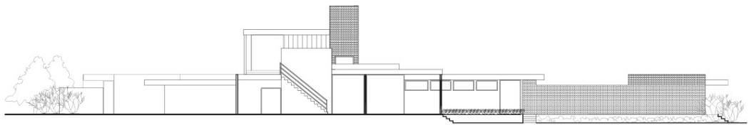
FACHADA SUR
